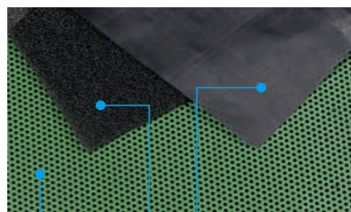
铝质喷涂面网+滤棉+网布 三层保护、防尘、防水面网
