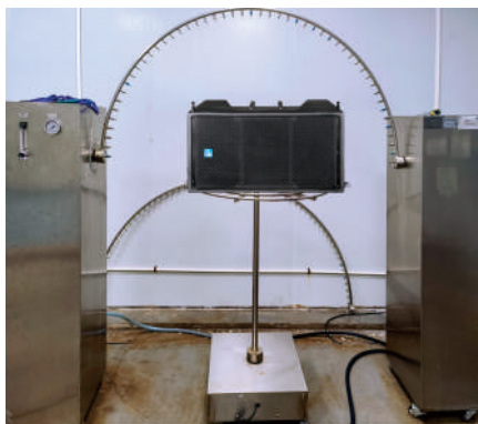
防水测试 Waterproof Test
