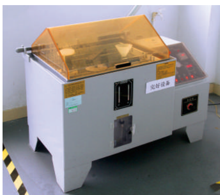
盐雾测试 Salt Spray Test
